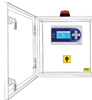
OUTER DOOR
